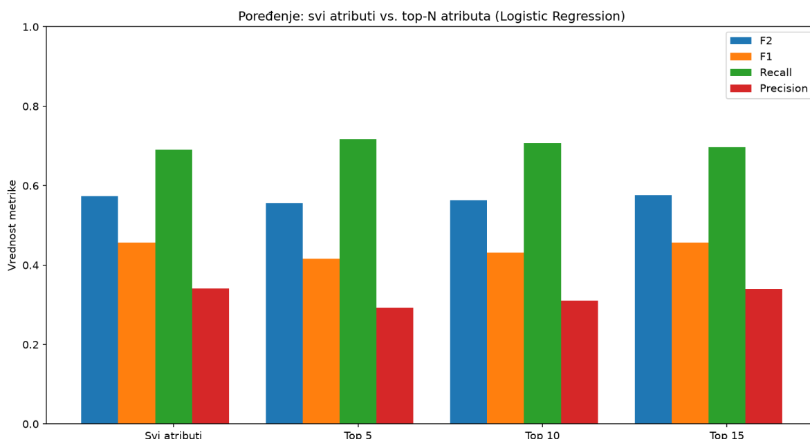
Slika 11: poređenje performansi modela kada su uključeni svi atributi i kada je uključeno top N atributa kod Logic Regression
