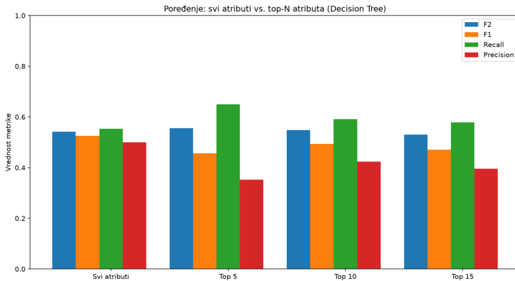
Slika 12: poređenje performansi modela kada su uključeni svi atributi i kada je uključeno top N atributa kod Decision Tree-a
