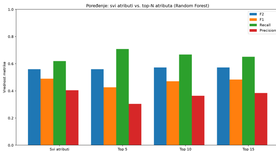
Slika 14: poređenje performansi modela kada su uključeni svi atributi i kada je uključeno top N atributa kod Random Foresta
