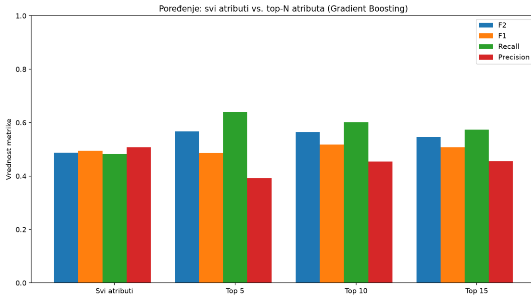
Slika 13: poređenje performansi modela kada su uključeni svi atributi i kada je uključeno top N atributa kod Gradient Boostinga
